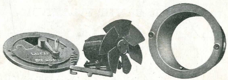
VENTILATEUR DÉMONTÉ
